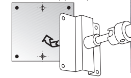
Abb. 7: MS-KGH Kugelgelenkhalterung
